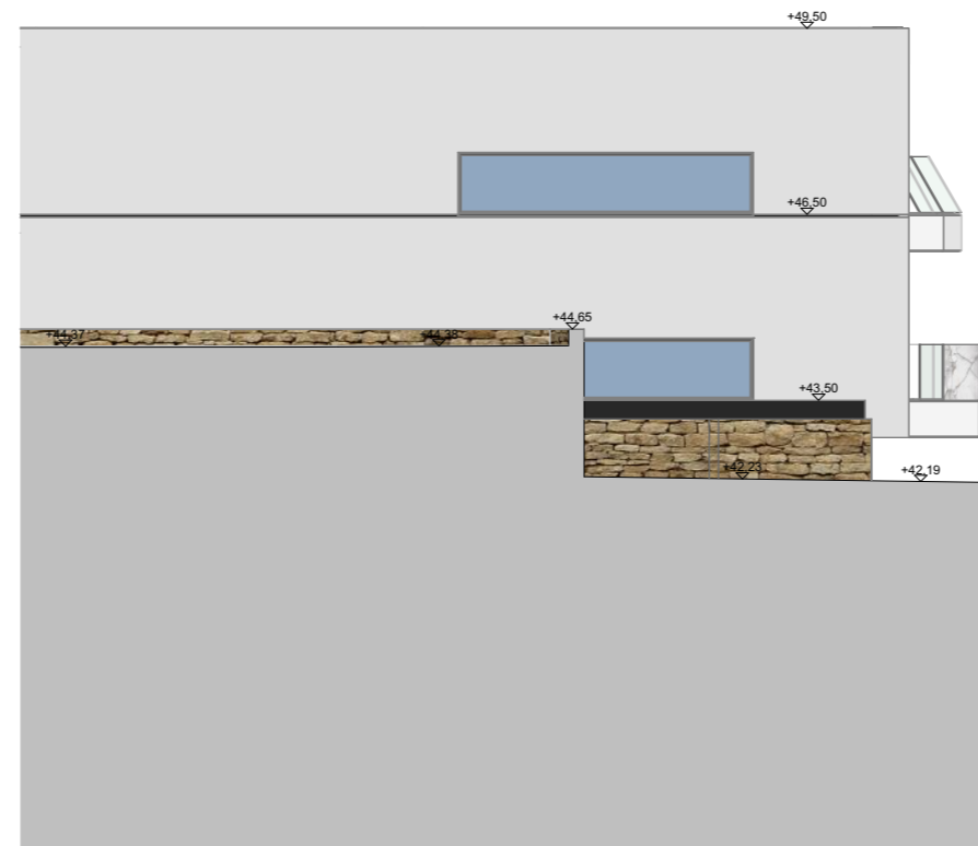
Alçado tardoz
