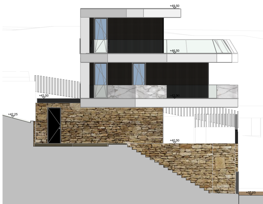
Alçado lateral
