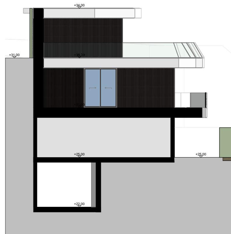
Alçado lateral
